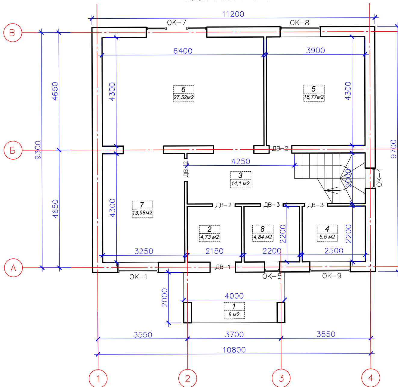
План 1-ого этажа
