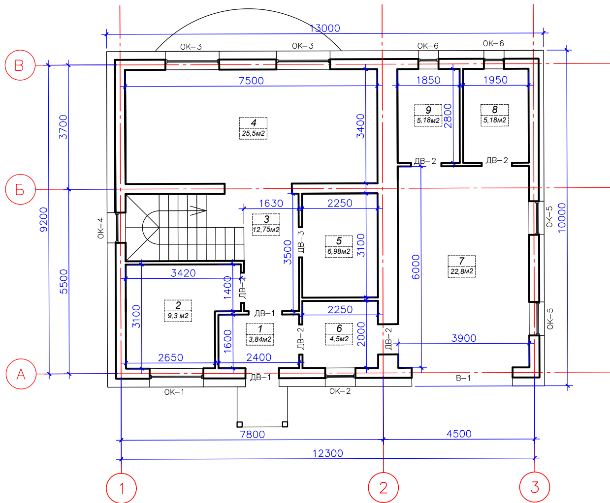
План 1-ого этажа
